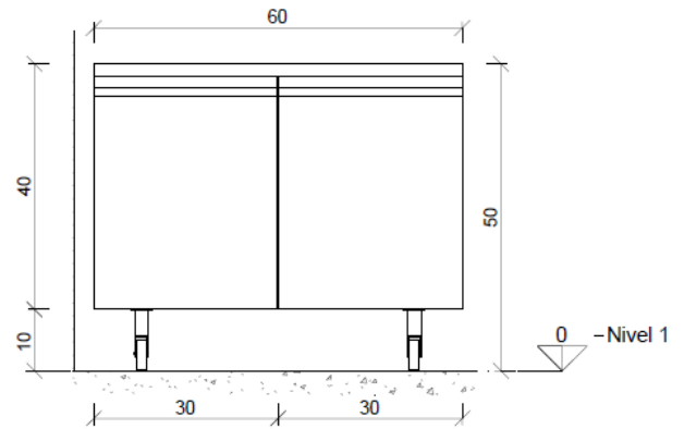
Gabinete impresora M4 - Elevación 1 1:10
