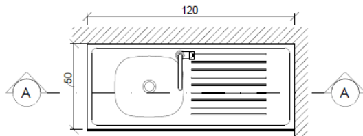
Lavaplatos M3 1:20
