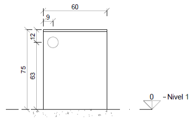
Escritorio M1 Elevación 3 1:20
