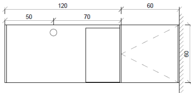
Escritorio M1 1:20
