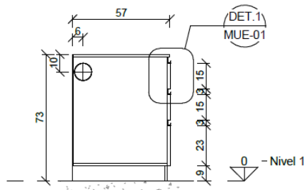
Gabinete Tipo - Elevación 1 1:20
