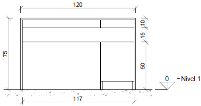
Escritorio M2 Elevación 2 1:20
