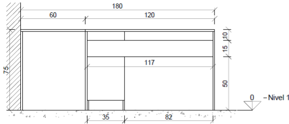
Escritorio M1 Elevación 2 1:20
