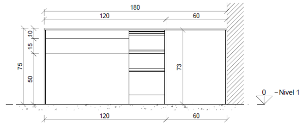
Escritorio M1 Elevación 1 1:20
