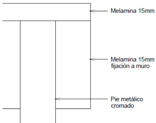
Meson M5 - Detalle 3 1:2
