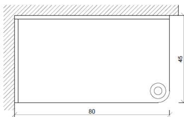
Meson M5 - planta 1:10
