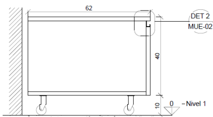
Gabinete impresora M4 - Elevación 2 1:10
