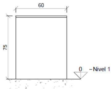
Escritorio M1 Elevación 4 1:20
