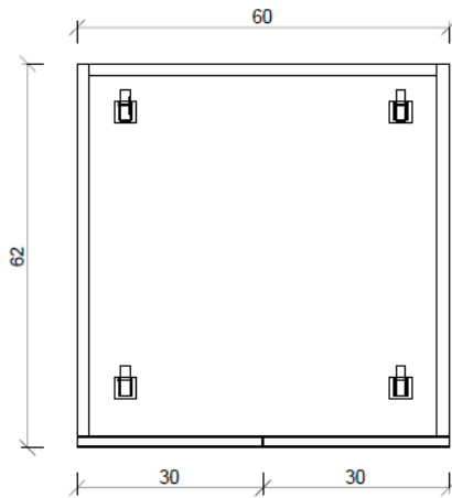
Gabinete impresora M4 - Planta 1:10
