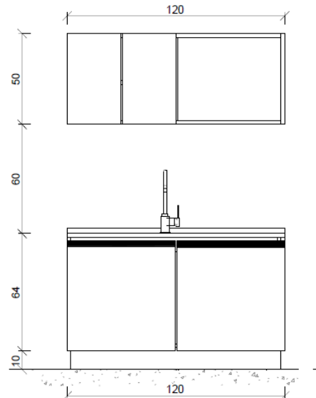
Lavaplatos M3 - Elevación 1 1:20
