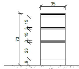
Gabinete Tipo - Elevación 2 1:20
