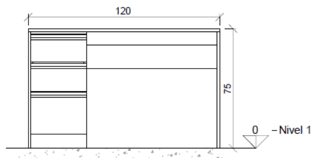
Escritorio M2 Elevación 1 1:20
