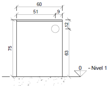
Escritorio M2 Elevación 4 1:20
