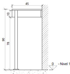
Meson M5 - Elevación 1 1:15
