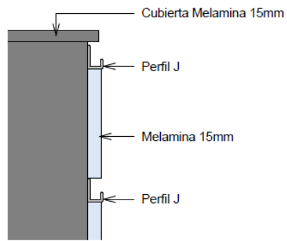
Gabinete Tipo - Detalle 1 Perfil J 1:5
