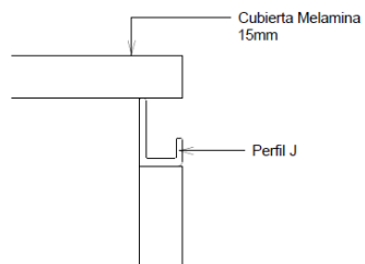
Gabinete impresora M4 - Detalle 2 1:2
