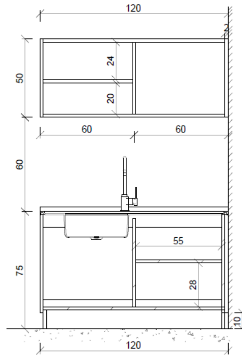
Lavaplatos M3 - Corte A-A 1:20
