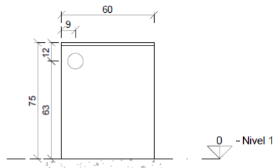
Escritorio M1 Elevación 3 1:20
