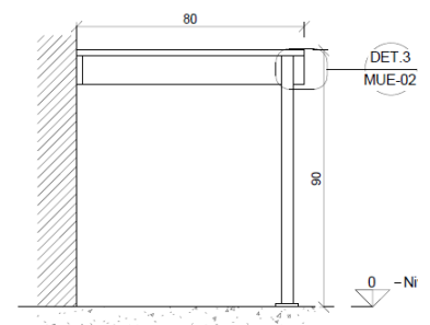
Meson M5 - Elevación 2 1:15
