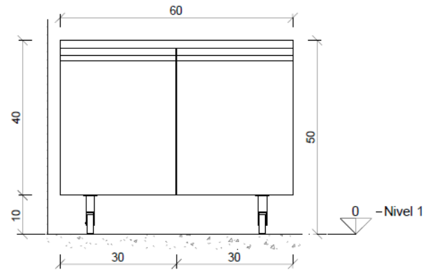
Gabinete impresora M4 - Elevación 1 1:10
