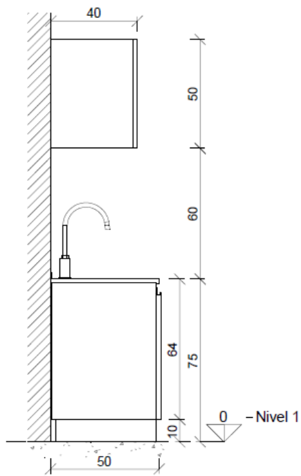
Lavaplatos M3 - Elevación 2 1:20
