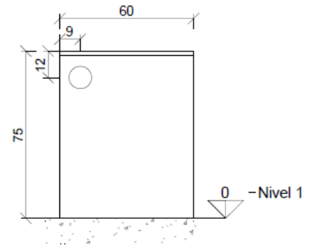
Escritorio M2 Elevación 3 1:20
