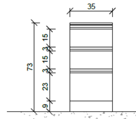
Gabinete Tipo - Elevación 2 1:20
