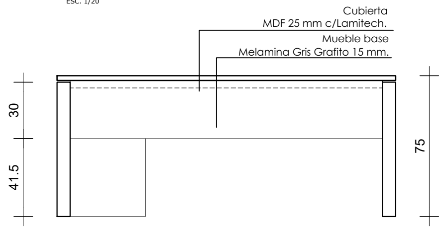
ELEVACIÓN POSTERIOR
