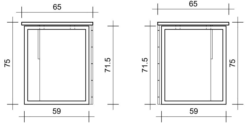
ELEVACIONES LATERALES
