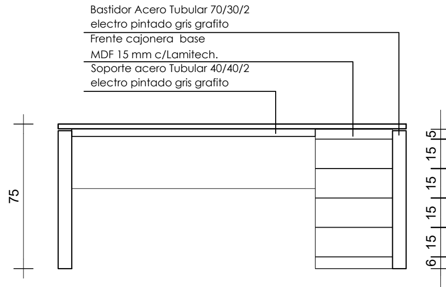
ELEVACIÓN FRONTAL
