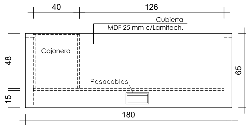
PLANTA
