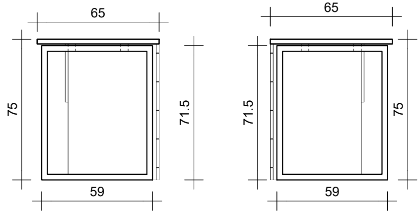
ELEVACIONES LATERALES
