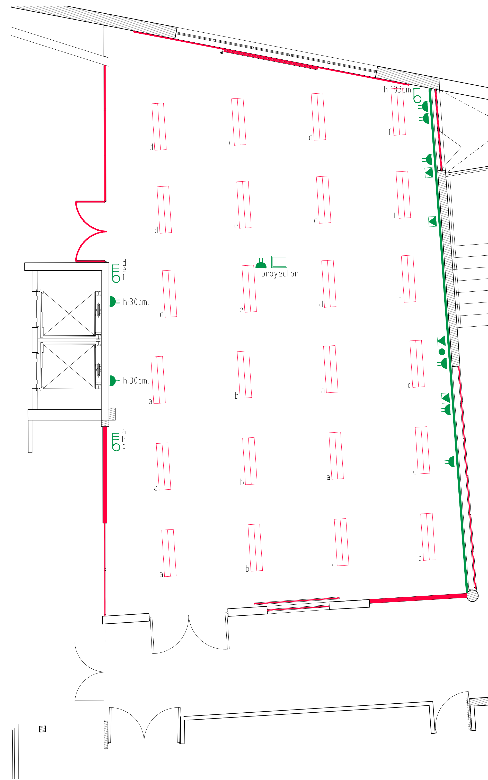
PLANTA PTOS. ELÉCTRICOS SITUACIÓN EXISTENTE escala 1/50
