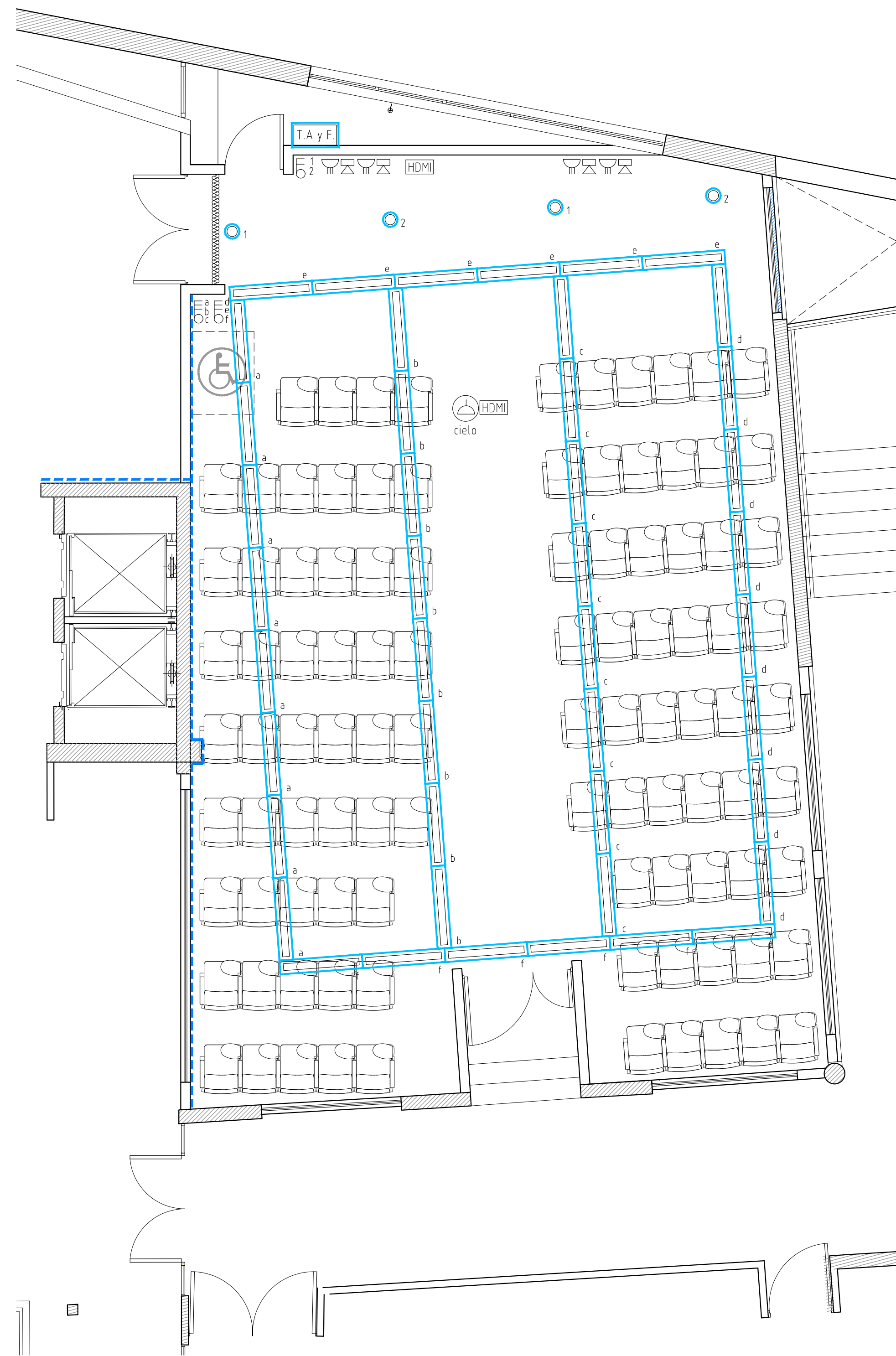
PLANTA PTOS. ELÉCTRICOS SITUACIÓN PROPUESTA escala 1/50
