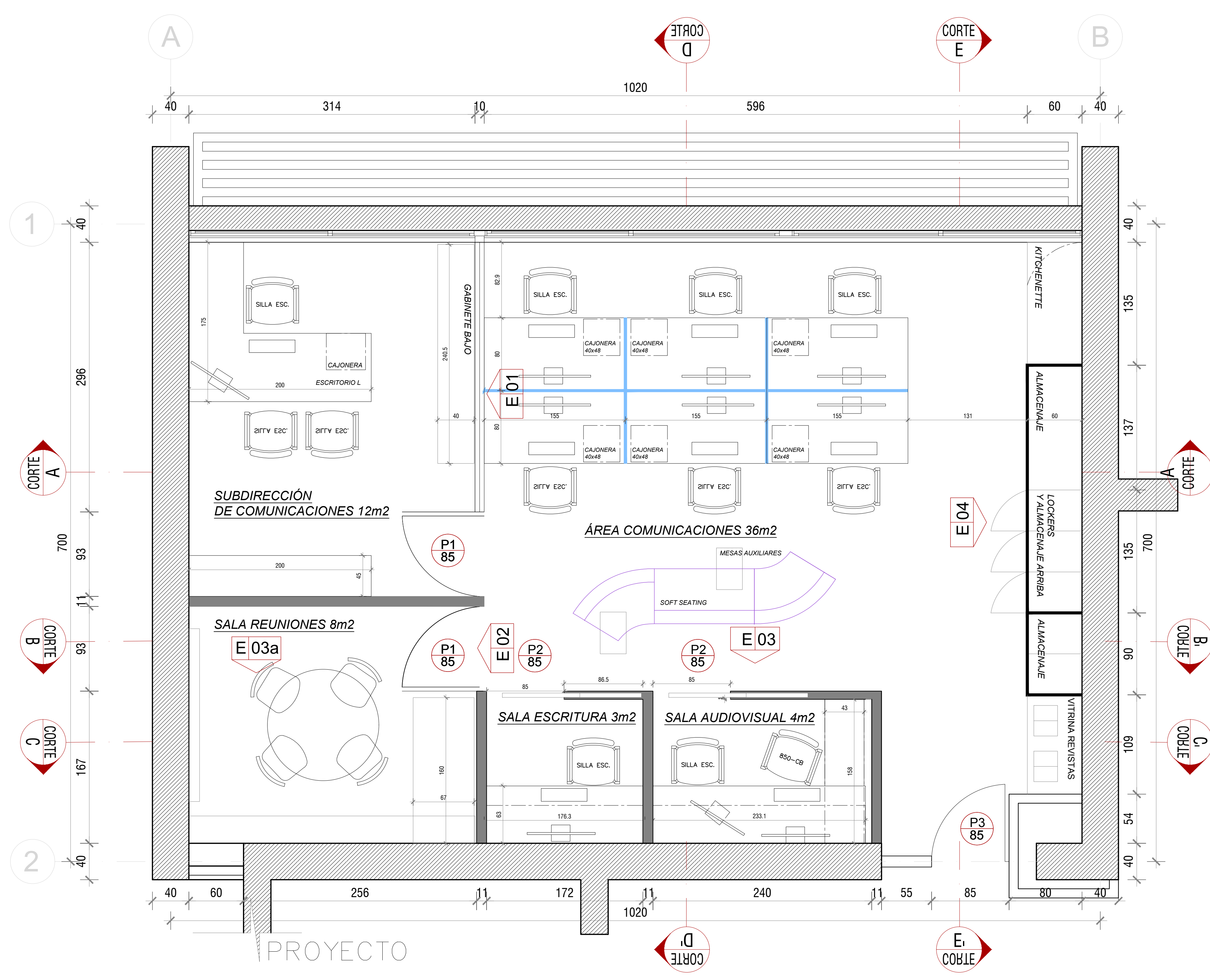
PLANTA PROYECTO ESC 1:40 PROYECTO COMUNICACIONES
