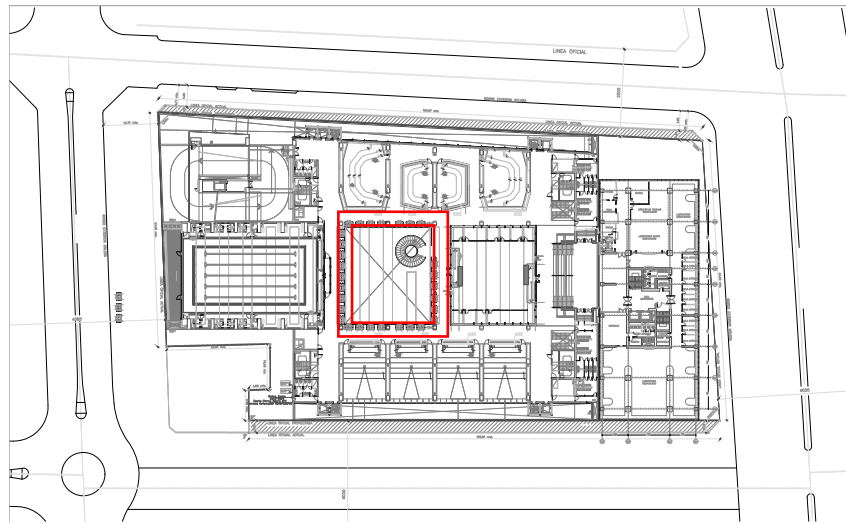
PLANTA SUBTERRÁNEO -1
